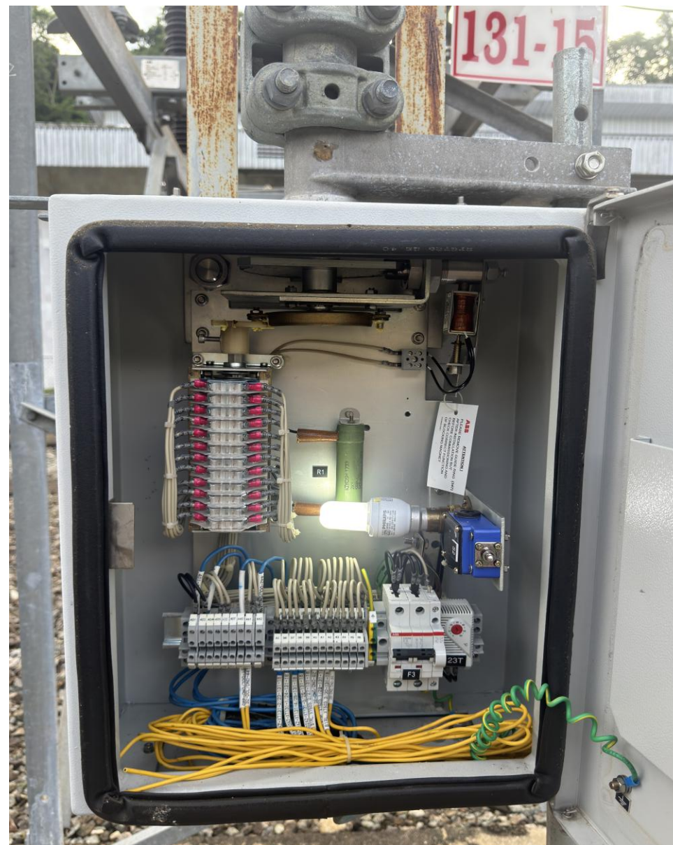
IX.8 – Tủ điều khiển DND 131-15
