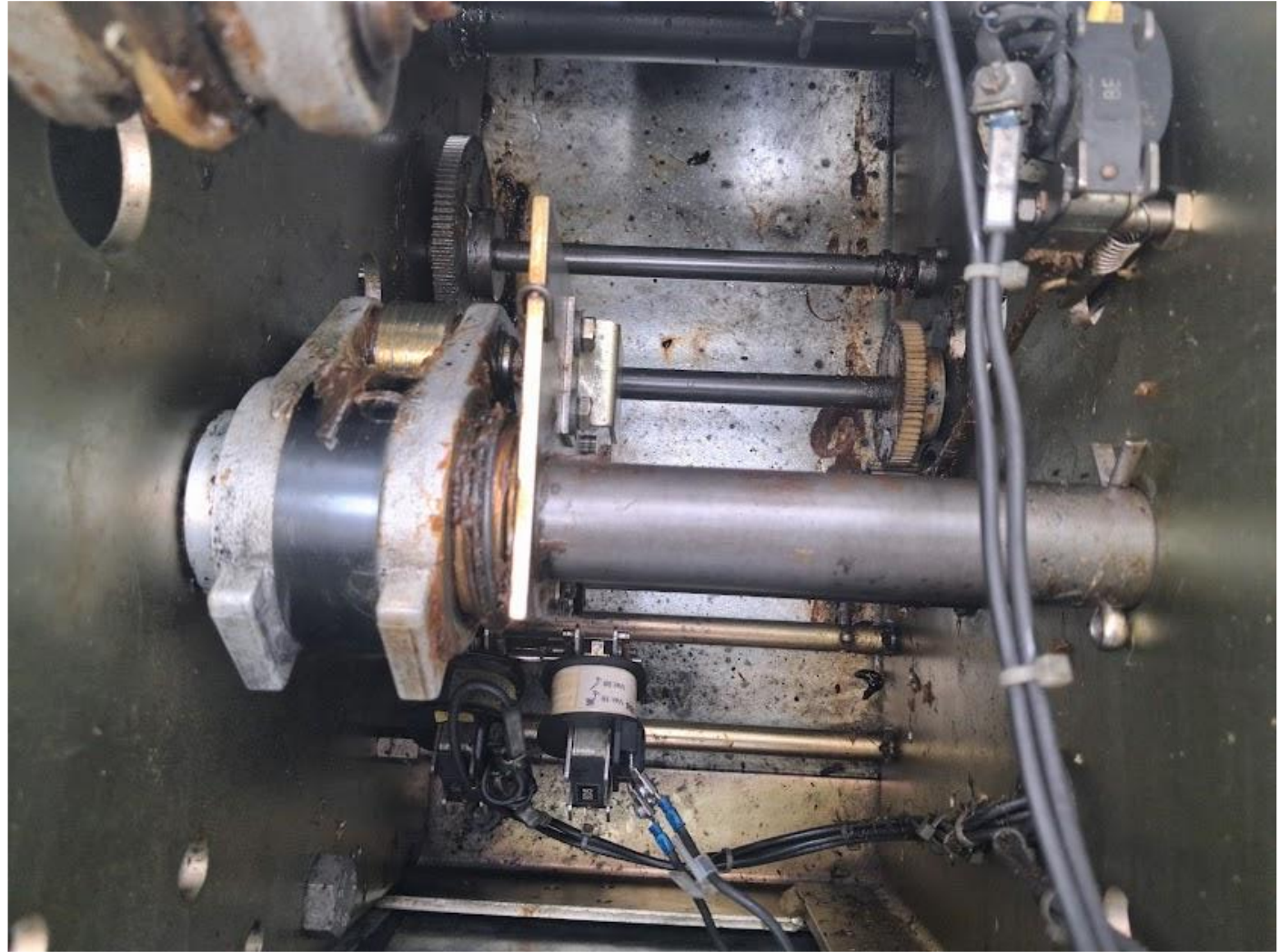
IX.4 - Truyền động bên trong MC 131
